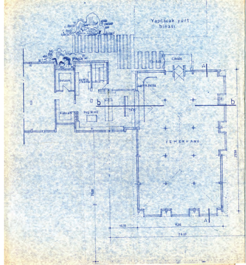
Yemekhane ve yurt binası planı. Hüsamettin Örüç arşivi
